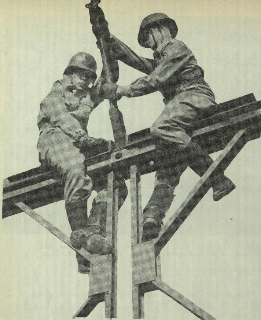
Dos Alféreces de Inge- nieros empleando la gata circular con el separador de paneles, con el fin de lograr ensamblar dos pa- neles.
