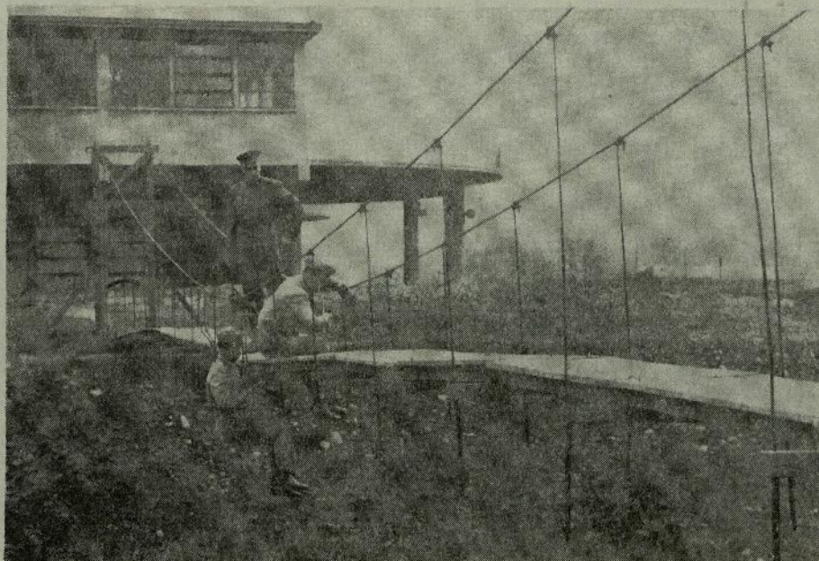
Alféreces de Ingenieros terminando la construcción de la Pasarela Suspendida sobre la futura piscina descubierta.
