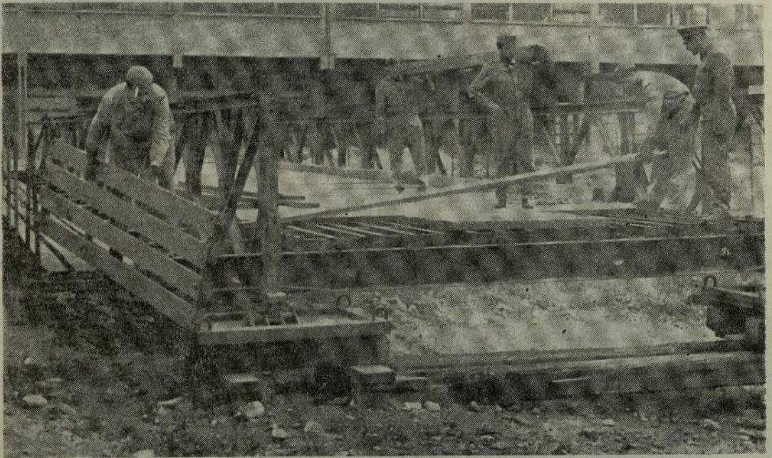
Construcción de una Sección de puente metálico tipo Bailey, por los Alféreces del Arma.
